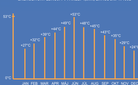
MAXIMÁLNE PRÍRASTKY TEPLoty V OBDOBÍ 1.10.2010 – 1.10.2011 ENERGETICKÝ ZDROJ: FV PANELY 1,0kW, LX ACDC/M+K 100L
