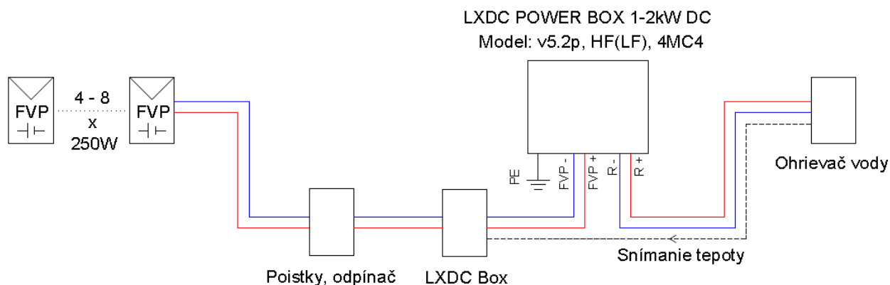
Bloková schéma zapojenia LXDC POWER BOX, variant č. 2
