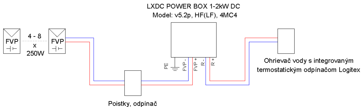
Bloková schéma zapojenia LXDC POWER BOX, variant č. 1
