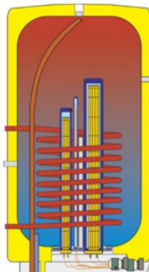
Bojler určený pre krby, pece a kotle
