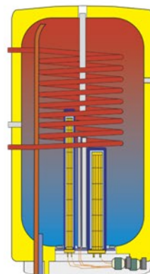
Špeciálny bojler určený pre plynové a elektrické kotle
