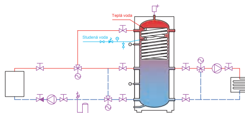
obr. 7 elektrická a hydraulická schéma zapojenia akumulacej nádrže NADO v11 s tepelným čerpadlom
