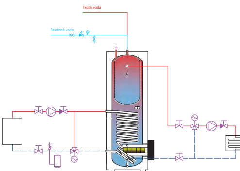
obr. 6 elektrická a hydraulická schéma zapojenia akumulacej nádrže NADO v2 s kotlom na tuhé palivá
